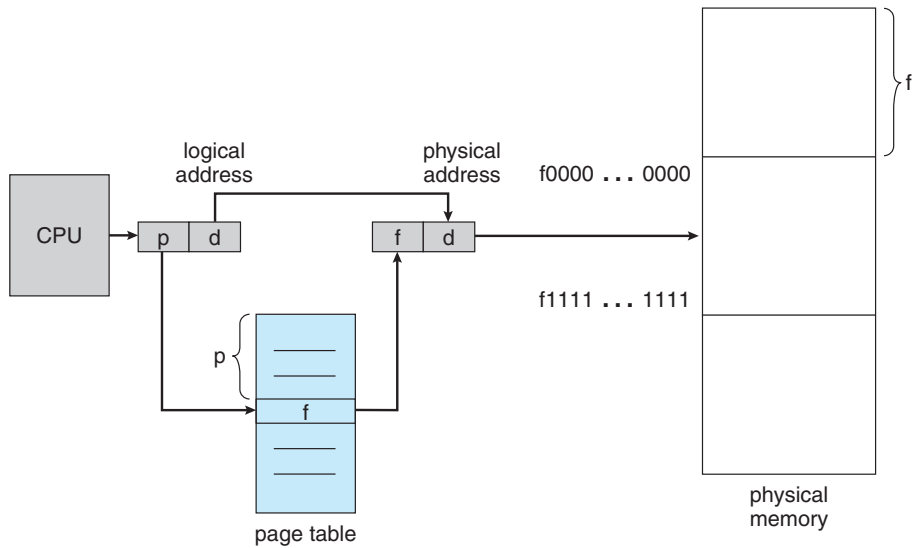
Figure 8.10 Paging hardware.
